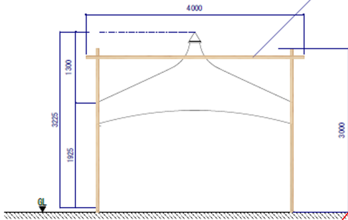
● 正面図
