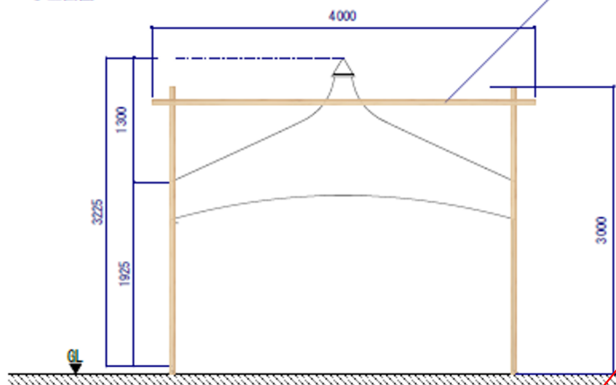
● 正面図
